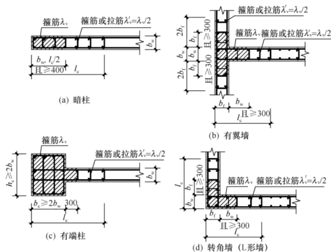
图 7.2.15 剪力墙的约束边缘构件
