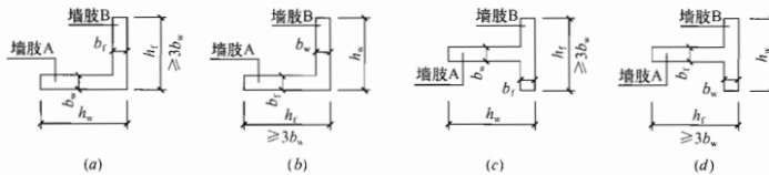
图 3.3.1-4 正交墙肢的互为翼墙 (a)、(c) 墙肢 B 为墙肢 A 的有效翼墙; (b)、(d) 墙肢 A 为墙肢 B 的有效翼墙
