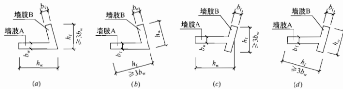
图 3.3.1-5 斜交墙肢的互为翼墙 (a)、(c) 墙肢 B 为墙肢 A 的有效翼墙; (b)、(d) 墙肢 A 为墙肢 B 的有效翼墙
