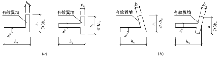
图 3.3.1-2 剪力墙的有效翼墙 (a) 正交墙肢；(b) 斜交墙肢
