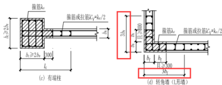
图 7.2.11 剪力墙的约束边缘构件
