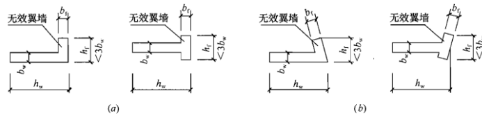
图 3.3.1-3 剪力墙的无效翼墙 (a) 正交墙肢; (b) 斜交墙肢
